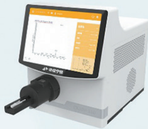
污水检测专用 便携式质谱仪
